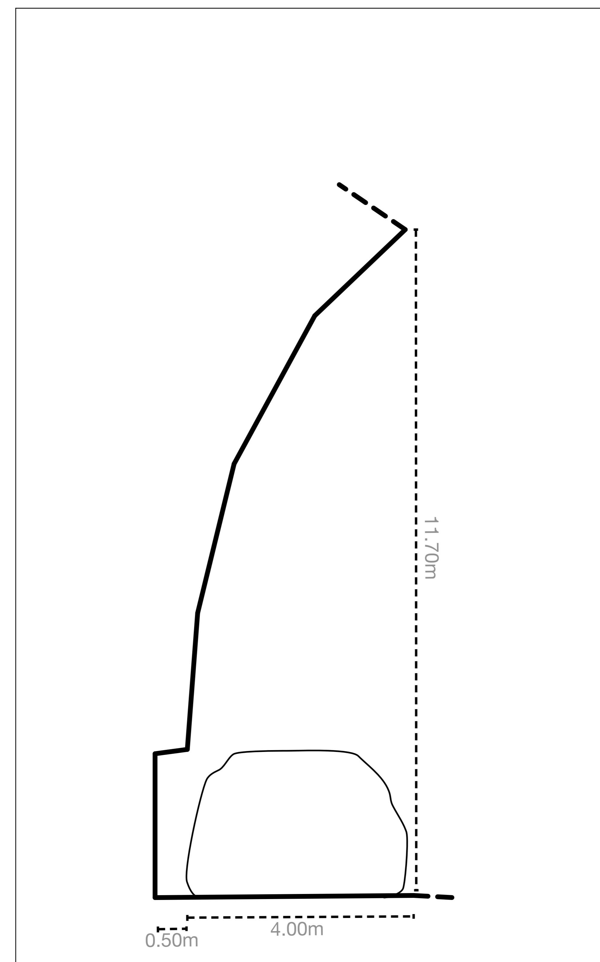
Poikkileikkaus B
