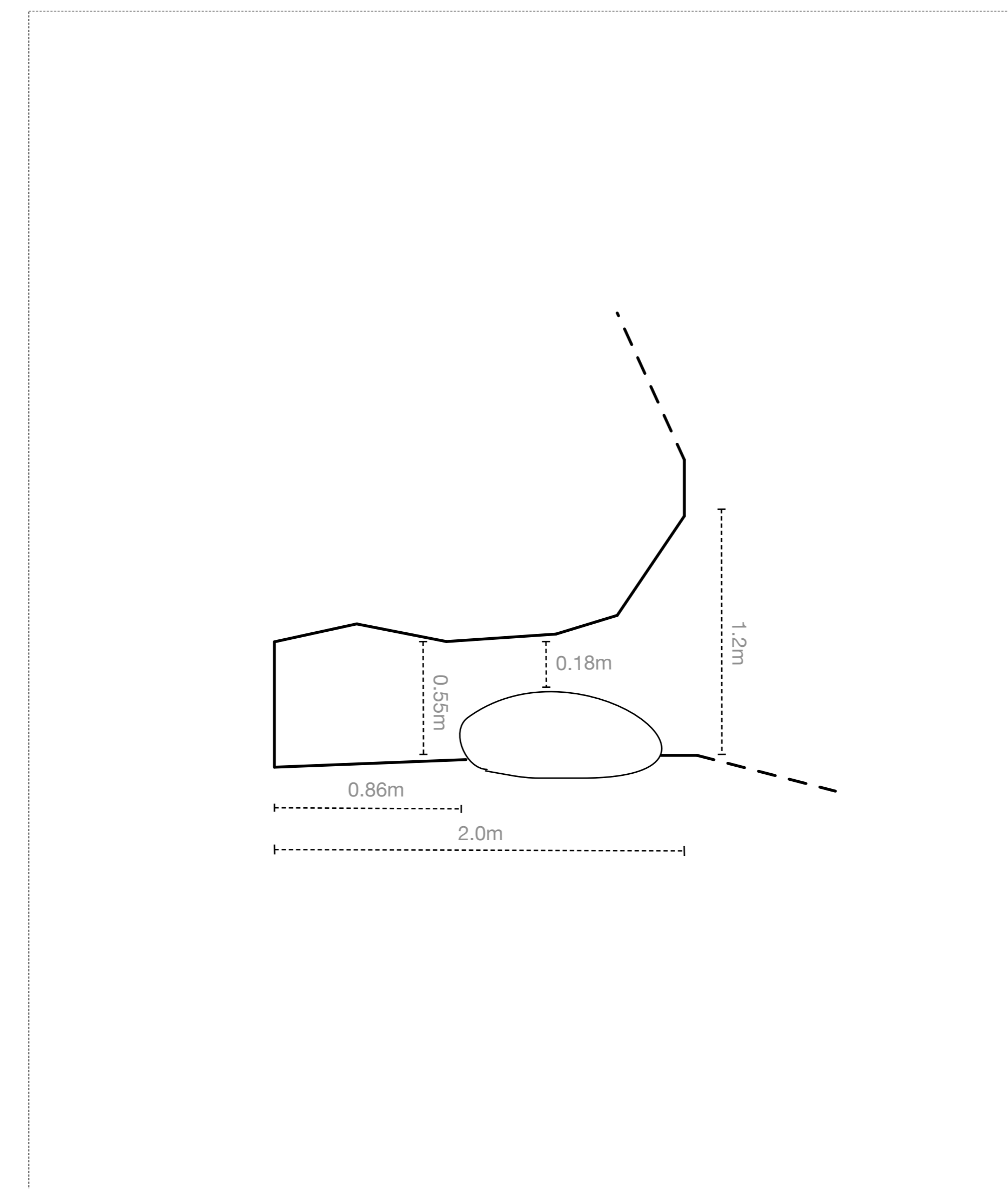
Poikkileikkaus B-B
