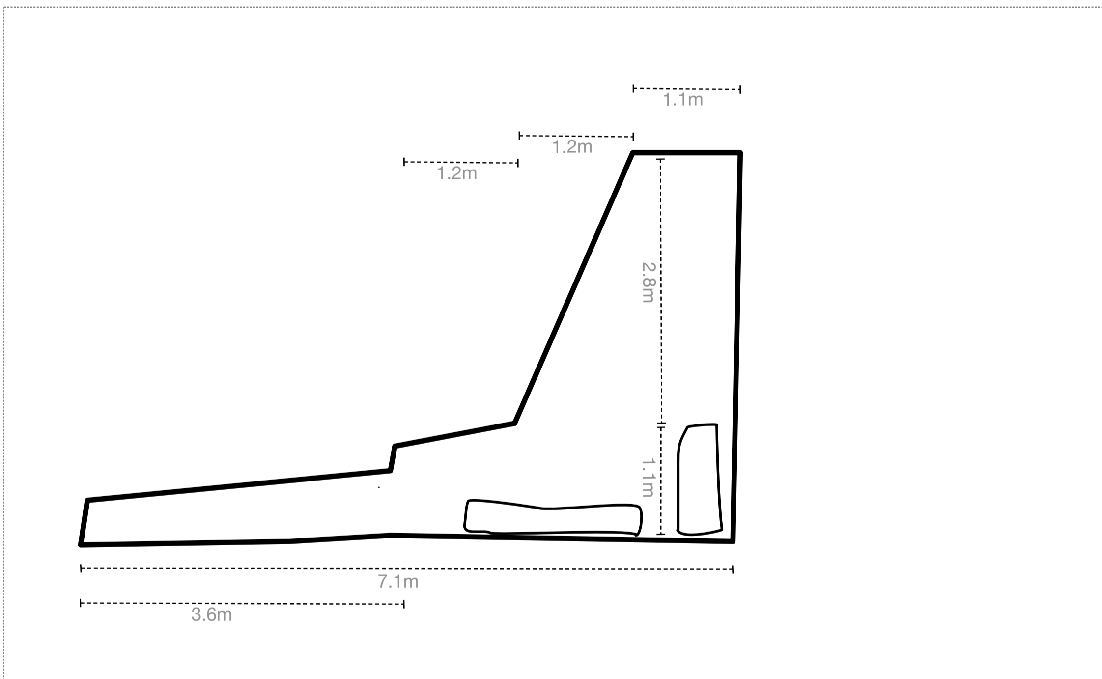
Poikkileikkaus A-A
