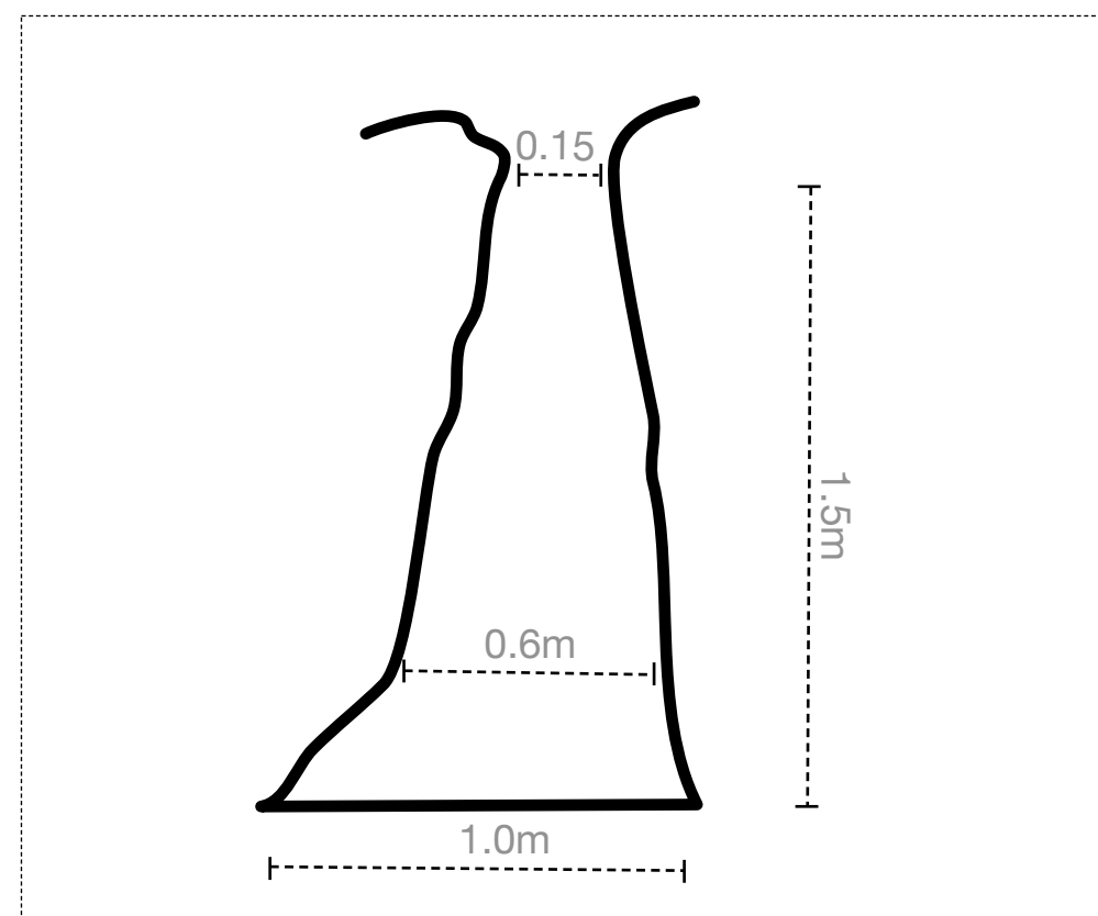
Sivuleikkaus A-A
