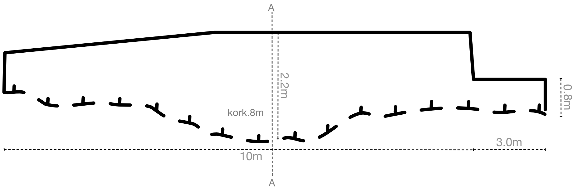
Poikkileikkaus A-A
